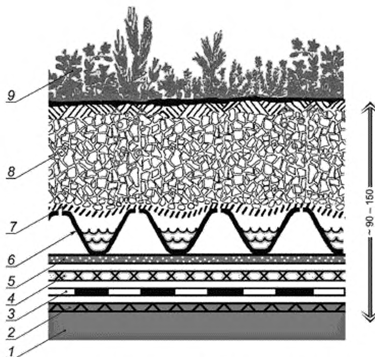
1 — несущая конструкция крыши; 2 — водоизоляционный слой; 3 — защитный слой; 4 — коррозийно-защитный слой; 5 — влагонакопительный слой; 6 — дренажный слой; 7 — фильтрующий слой; 8 — субстрат; 9 — растительный слой
