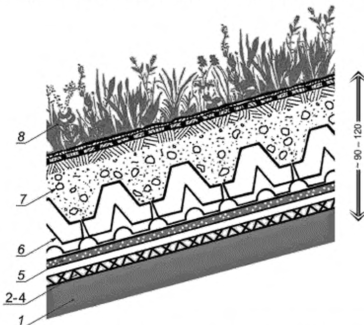
1 — несущая конструкция крыши; 2—4 — водонепроницаемый, корнесащитный слой «два в одном»; 5 — влагозащитный слой; 6 — дренажный слой; 7 — субстрат; 8 — растительный слой
