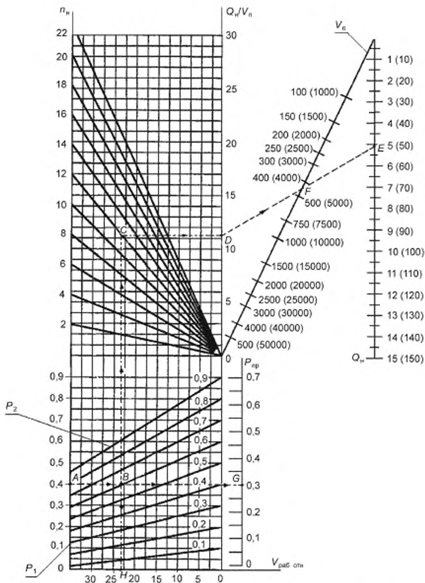
Рисунок Е.3 — Номограмма для определения объема пневмоцистерны
