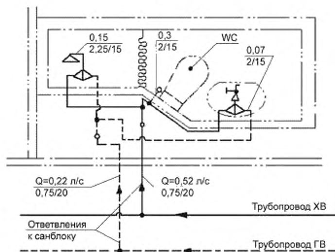
Рисунок Е.1 — Расчетная схема каютного санитарно-гигиенического блока
