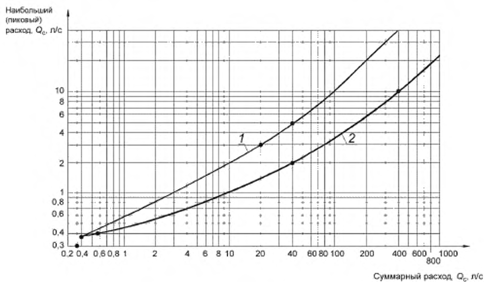
Рисунок Г.1 — График для определения наибольшего (пикового) расхода питьевой воды в зависимости от суммарного расхода воды
