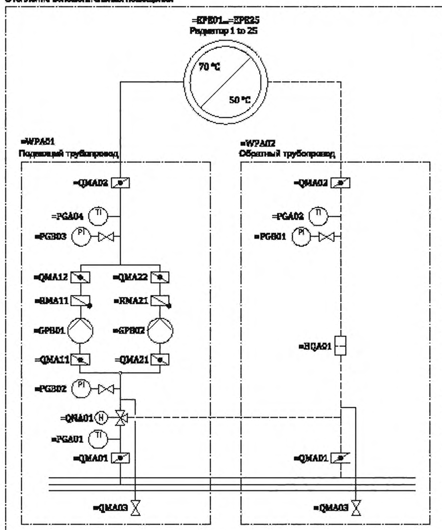
Рисунок В.17 — Принципиальная схема системы отопления
