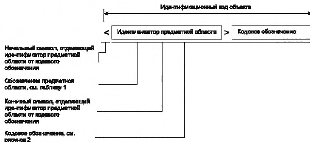
Рисунок 1 — Применение идентификатора предметной области
