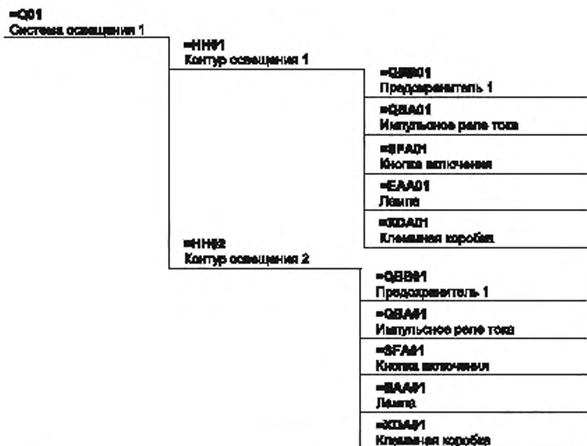
Рисунок В.22 — Древоидная функционально-ориентированная структура двух контуров освещения согласно рисунку В.21
