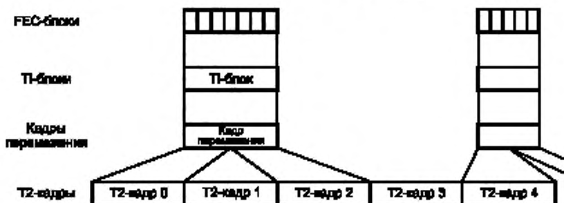
Рисунок 16 — Перемежение по времени для P_1 = 2 , I_{\text{JUMP}} = 2 , N_{T1} = 1
