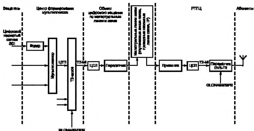
Рисунок 34 — Типовая структурная схема телевизионного вещания
