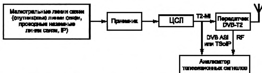
Рисунок 38 — Схема проведения измерений параметров сквозной передачи цифрового телевизионного сигнала на объекте вещания
