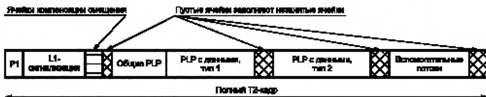
Рисунок 29 — Структура T2-кадра
