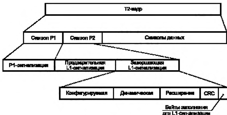
Рисунок 19 — Структура L1-сигнализации
