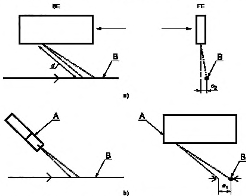
А — датчик; В — струна; SE — вид сбоку; FE — вид спереди, — — — — номинальное направление оси доплеровского пучка; — — — — действительное направление оси доплеровского пучка
