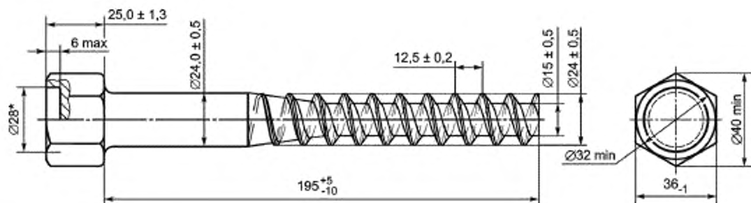
Конструкция Б, исполнение 2
