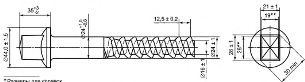
Рисунок 4 — Конструкция и основные размеры шурупа, используемого в рельсовых креплениях с железобетонным подрельсовым основанием
