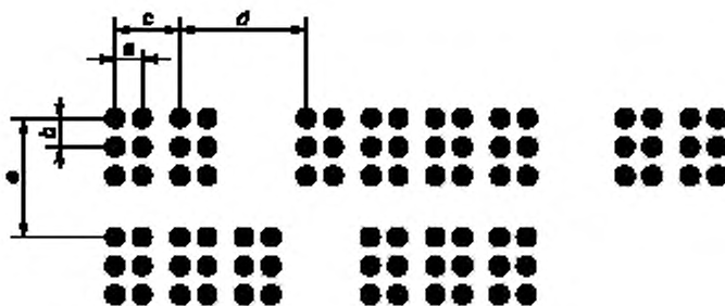
Рисунок 2 — Схема размеров рельефно-точечного шрифта Брайля
