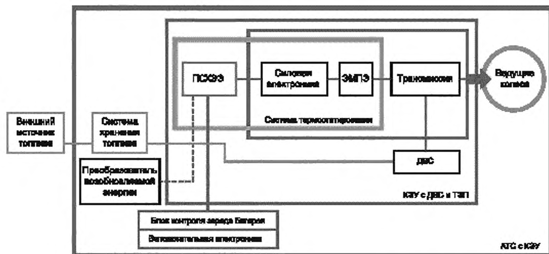
Рисунок А.2 — Возможная схема автомобильного транспортного средства с комбинированной энергетической установкой параллельного типа без возможности внешней зарядки
