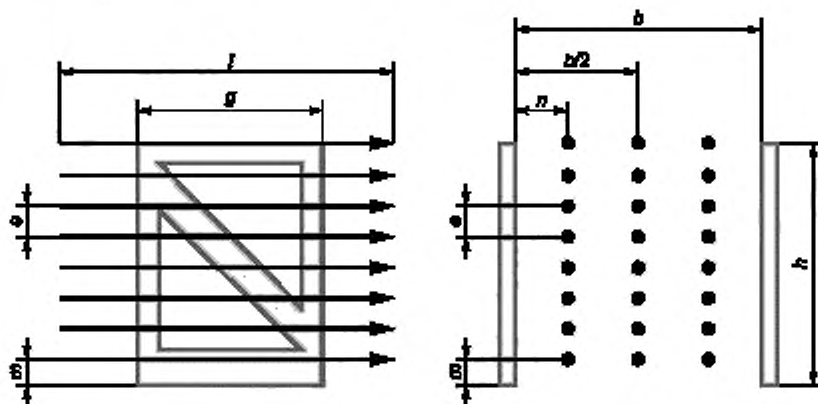
b — ширина ворот; g — расстояние между горизонтальными плоскостями прохода; g — ширина антенны; l — расстояние прохода; h — расстояние до верхней границы области обнаружения; m — расстояние до нижней границы области обнаружения; n — расстояние от плоскости антенны до первых точек измерений.
