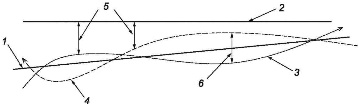
1 — линия A—B; 2 — постоянная линия на поверхности земли; 3 — предыдущая траектория перемещения репрезентативной точки машины; 4 — следующая траектория перемещения репрезентативной точки машины; 5 — относительные измерения позиции отслеживающим датчиком; 6 — относительная XTE
