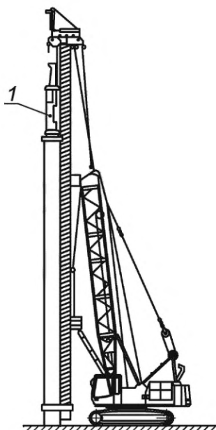
Рисунок 27 — Сваезабивное оборудование
