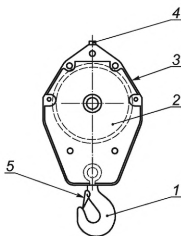
Рисунок 20 — Крюк в сборе
