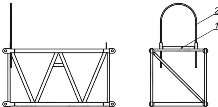
Рисунок 19 — Нижняя секция стрелы
