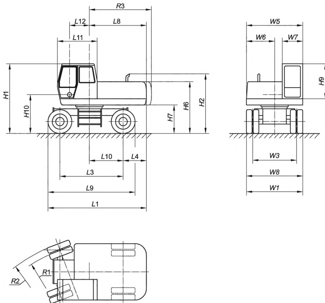
Рисунок 4 — Размерные характеристики базовой машины. Колесный экскаватор
