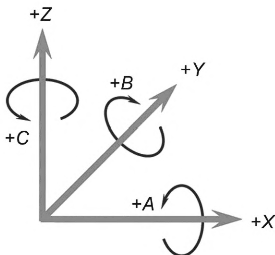
Рисунок А.1.3 — Правило «правой руки» для определения положительного направления вращения относительно начальной ориентации построения
