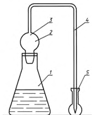
Прибор для отгонки и поглощения мышьяка
