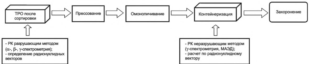
Рисунок Б.3 — Производственно-технологическая цепочка обращения с прессуемыми РАО АС с указанием этапов проведения РК
