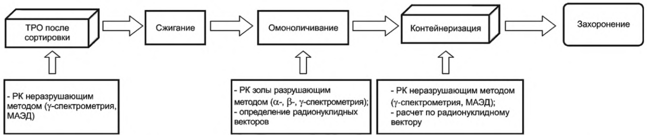
Рисунок Б.2 — Производственно-технологическая цепочка обращения с сжигаемыми РАО АС с указанием этапов проведения РК
