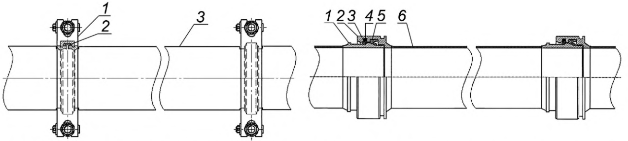
1 — соединительный замок; 2 — уплотнительная манжета; 3 — труба СРТ
