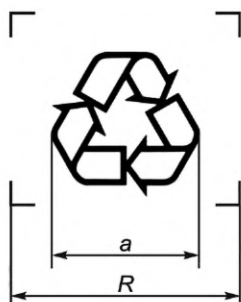
Рисунок Г.2 — Размеры символа переработки
