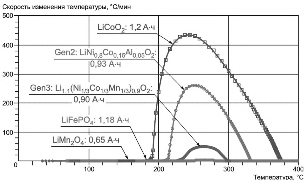
Рисунок А.2 — Скорость возрастания температуры различных катодных материалов при тепловом разгоне
