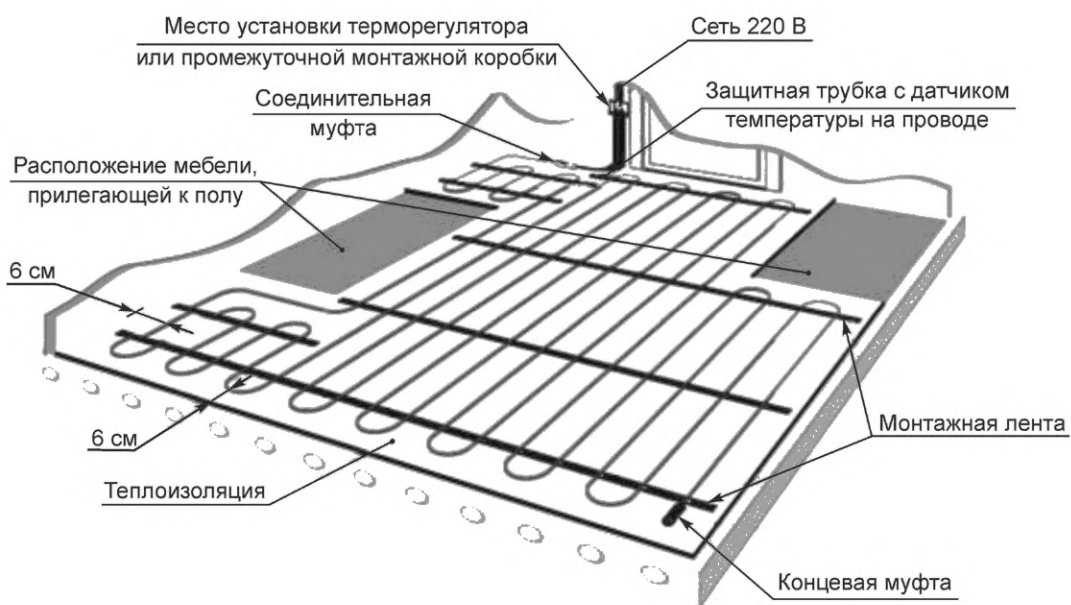
Рисунок Г.2 — Схема укладки кабельной нагревательной секции в помещении
