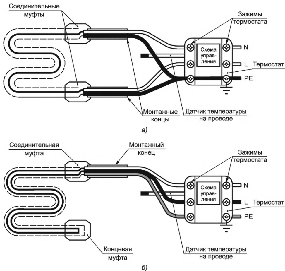
а) — на основе одножильного нагревательного кабеля; б) — на основе двухжильного нагревательного кабеля
