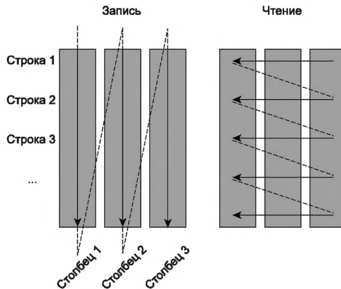
Рисунок 7 — Схема битового перемешивания для 8PSK при скорости кодирования 3/5
