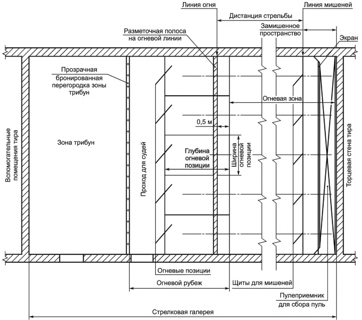
Рисунок А.1 — Стрелковая галерея крытого тира (пример компоновки с зоной трибун)
