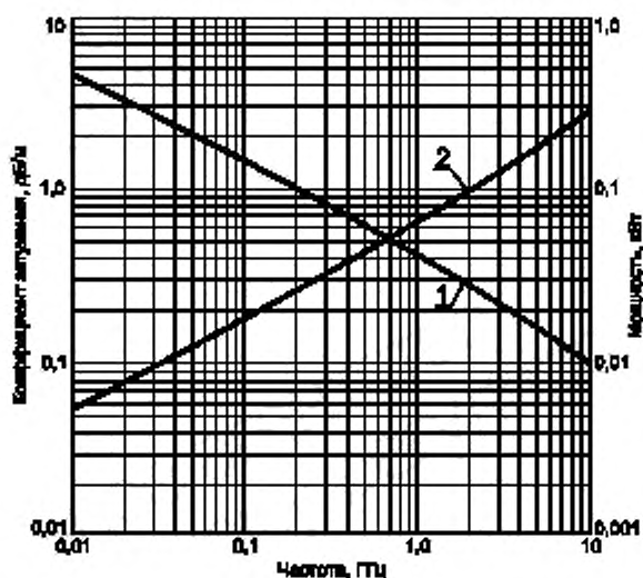
Частотные зависимости
