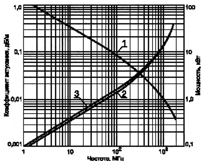
Частотные зависимости
