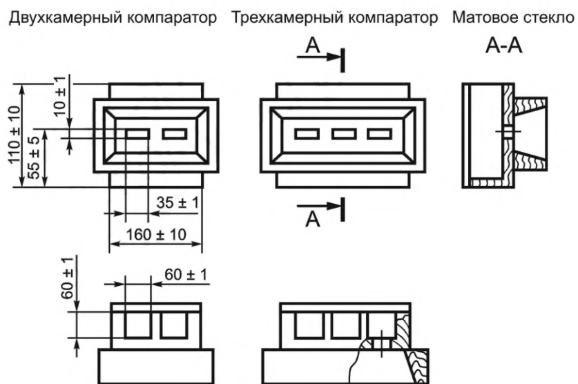
Рисунок А.1 — Компаратор
