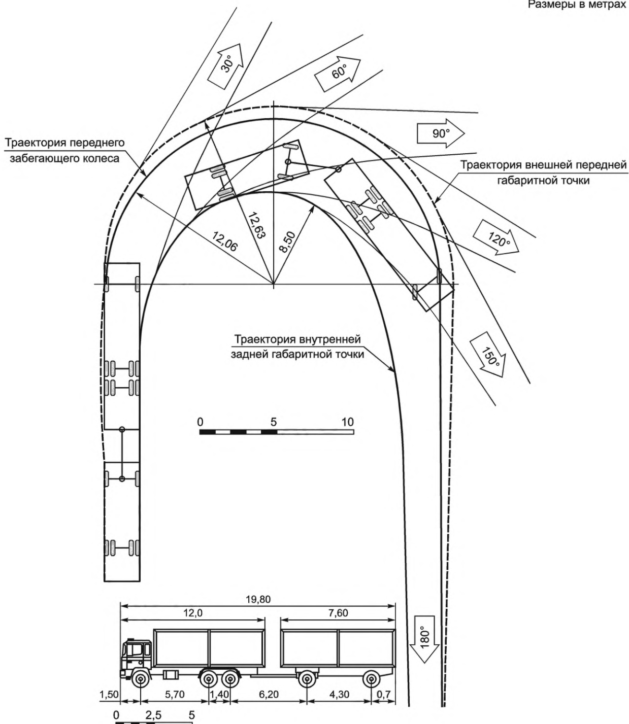
Рисунок 8 — Коридор, занимаемый расчетным автомобилем, равный 4,13 м
