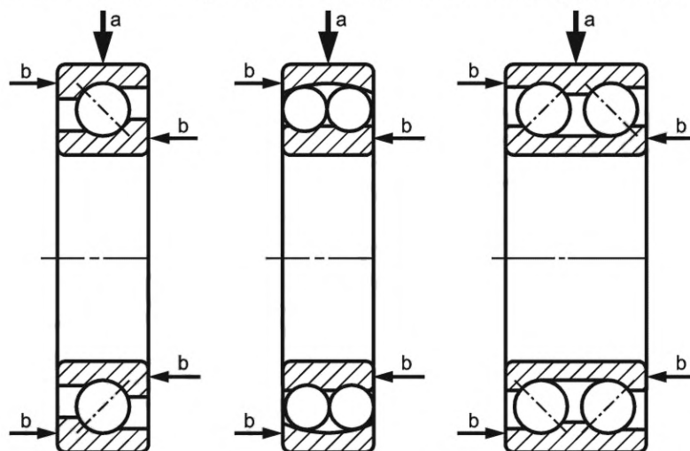
a — расположение и направление преобразователя; b — направление осевой нагрузки
