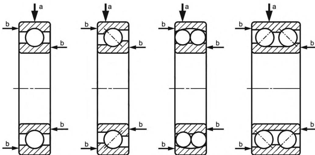
a — положение и направление преобразователя; b — направление осевой нагрузки
