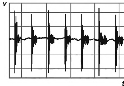
Рисунок 2 — Пример пульсации во временной области
