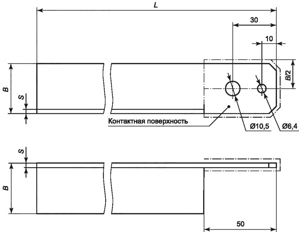
Рисунок 1 — Стойка заземления
