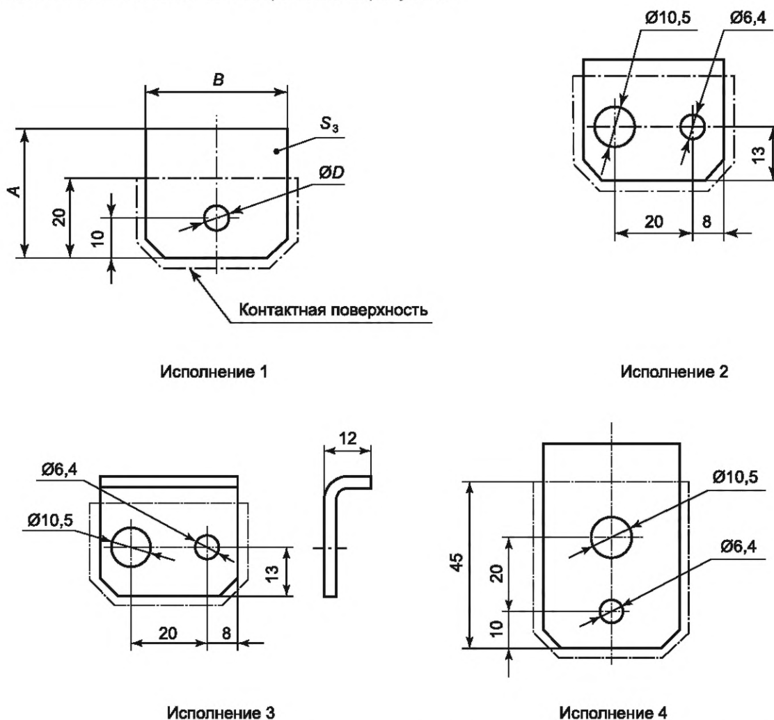
Рисунок 2 — Планки заземления
