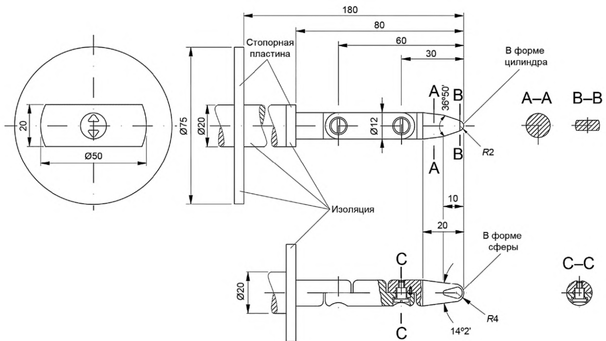
Рисунок 2 — Шарнирный зонд
