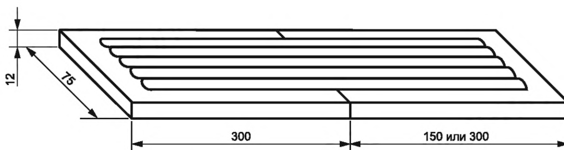
Рисунок 1 — Испытательный образец
