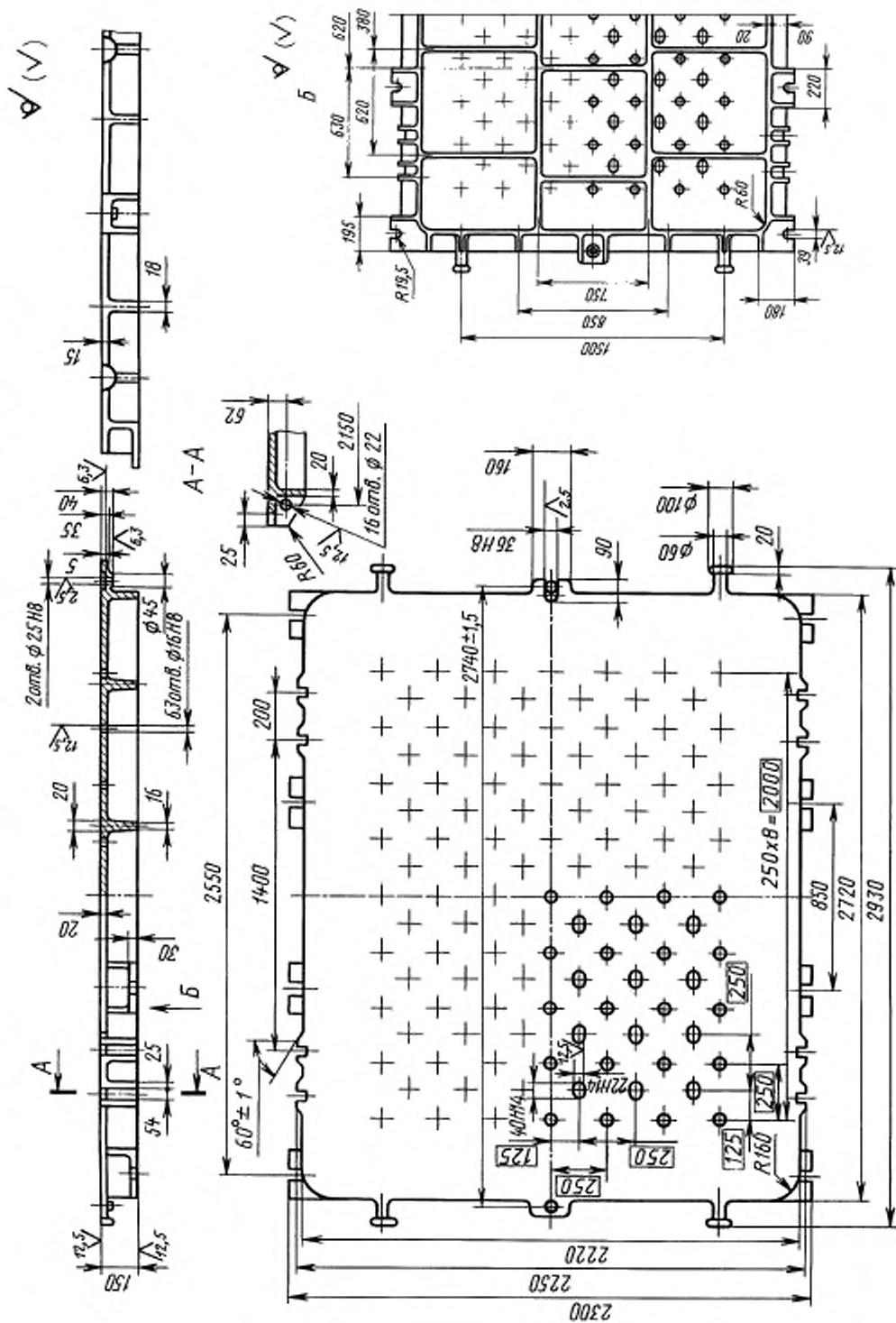
Пример 2 Стальная координатная модельная плита для машинной формовки под опоку размерами в свету 2500 × 2000 мм
