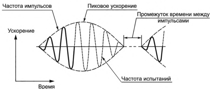
Рисунок 1 — Синусоидальные импульсы
