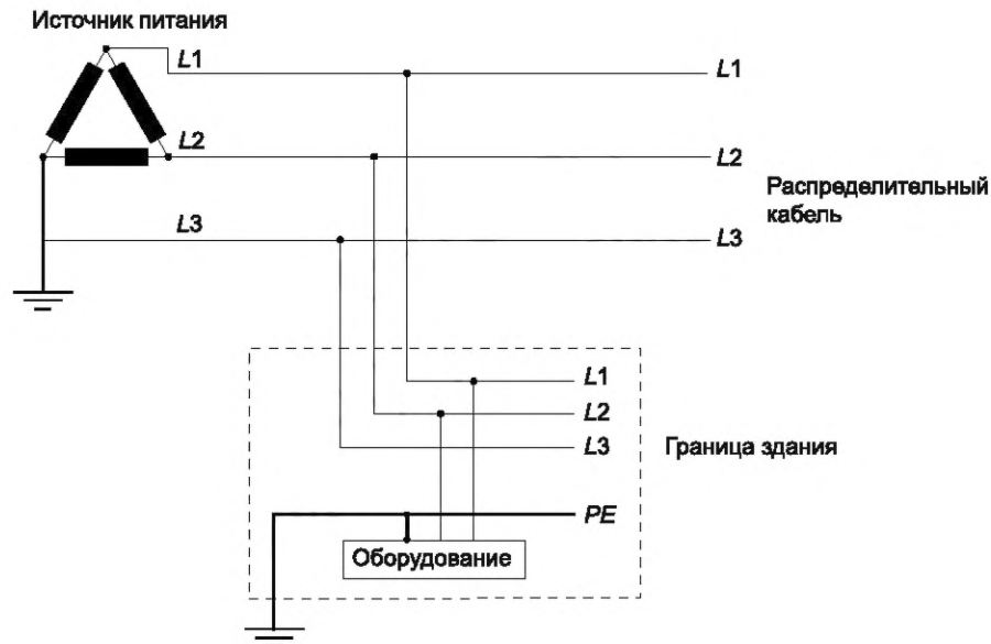
Рисунок I.6 — Пример трехфазной системы энергообеспечения TT
