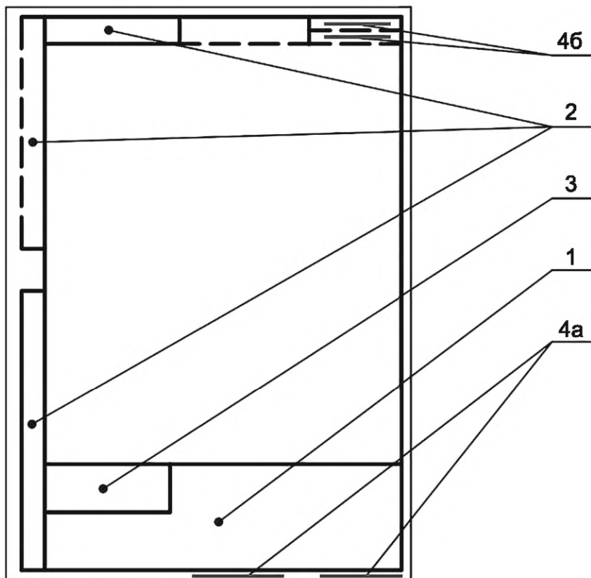
Рисунок В.1 — Размещение основной надписи для формата А4
