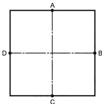
Рисунок 1 — Измерение расстояний на испытуемых пробах квадратной формы
