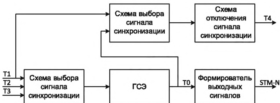
Рисунок 1 — Схема распределения сигнала синхронизации в мультиплексоре СЦИ
