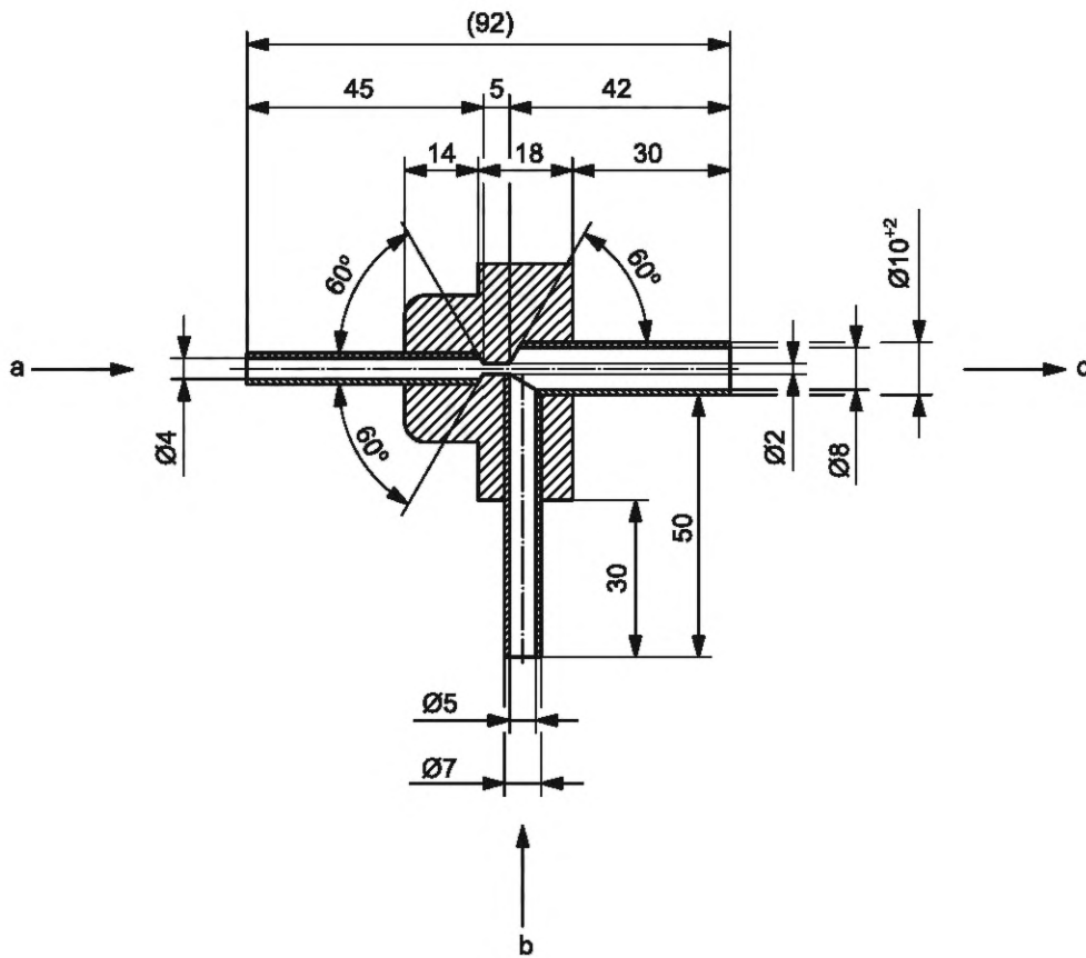
Рисунок 4 — Инжектор пыли
