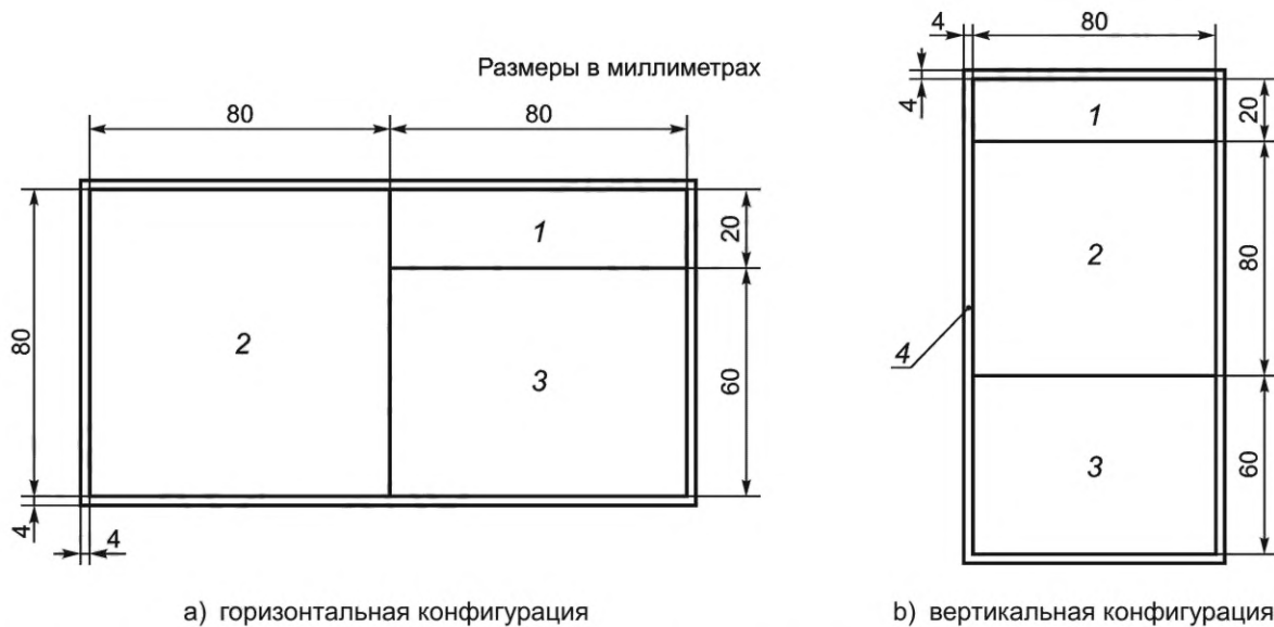
Рисунок 12 — Рекомендуемые размеры. Двухпанельный формат
