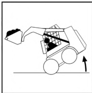
Рисунок А.42 — Опрокидывание машины. Перегруз. Минипогрузчик
