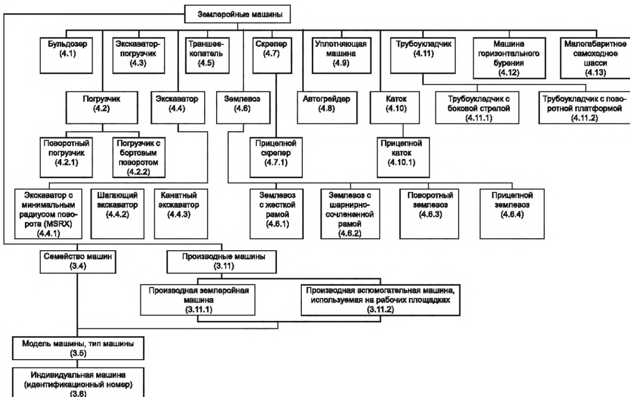
Рисунок А.1 — Схема идентификации машин
