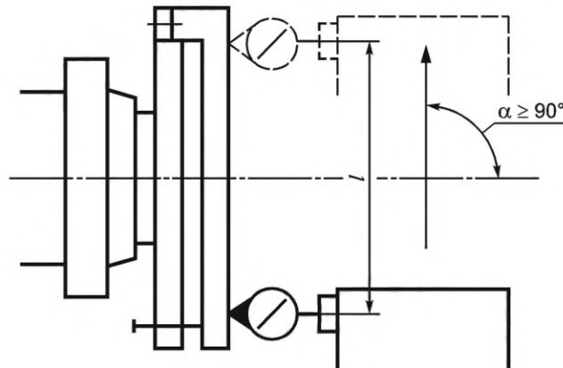
Рисунок 23 — Схема измерения отклонений от перпендикулярности направления перемещения рабочего органа к оси вращения шпинделя
