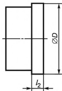
Рисунок 28 — Образец-изделие для проверки круглости
