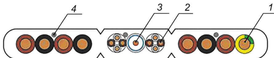
1 — основные жилы; 2 — элемент передачи сигналов (скрученные четверки); 3 — элемент передачи сигналов (коаксиальный элемент); 4 — вспарывающая нить
