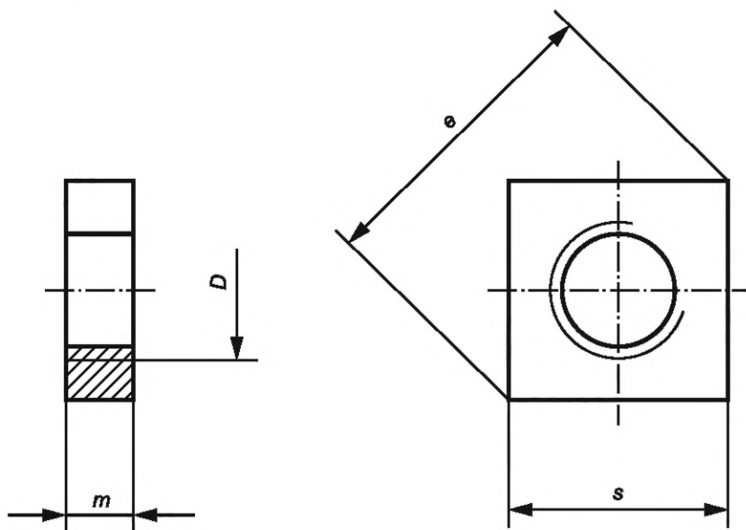
Рисунок 1 — Квадратные гайки
