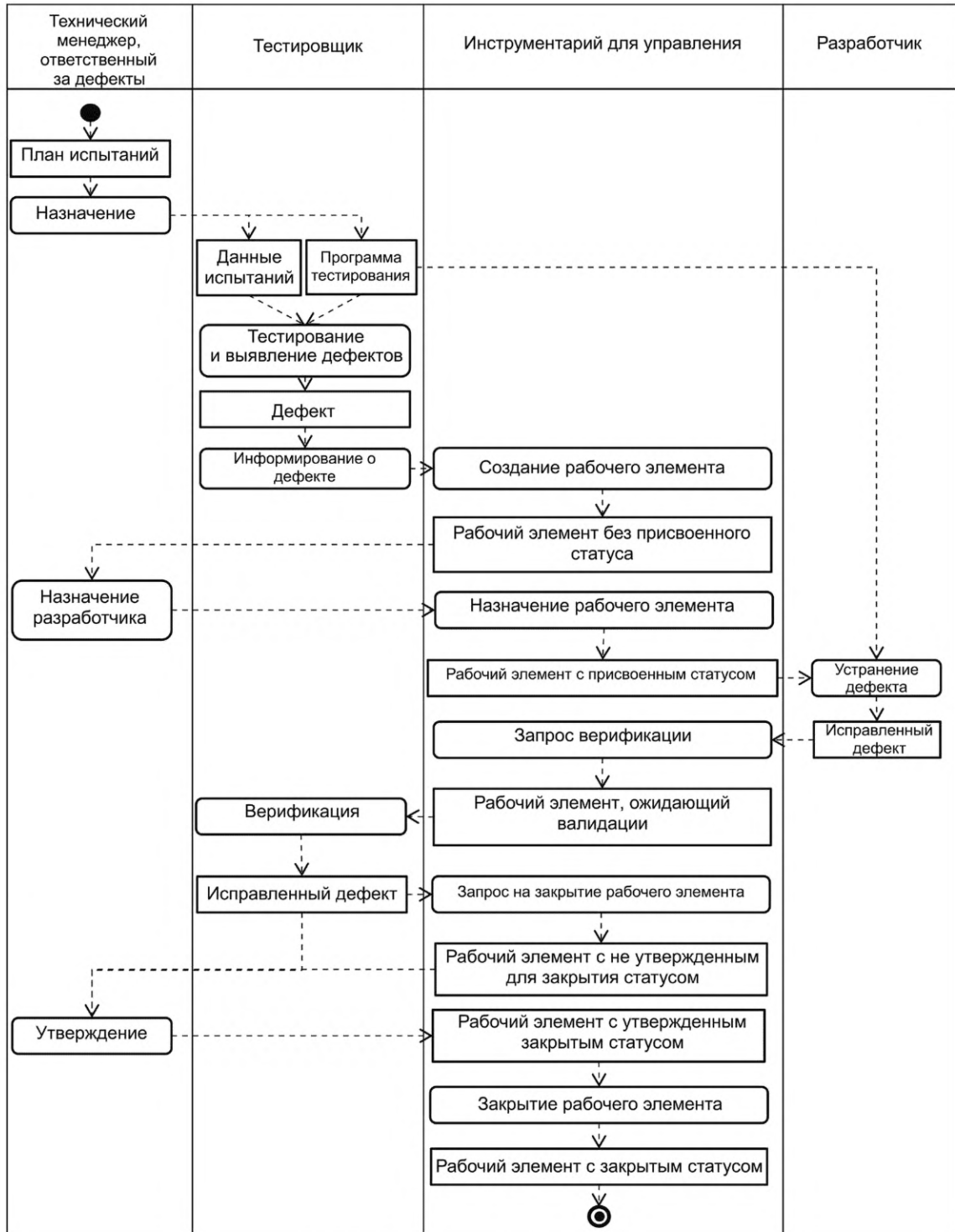
Рисунок 3 — Схема деятельности по управлению дефектами
