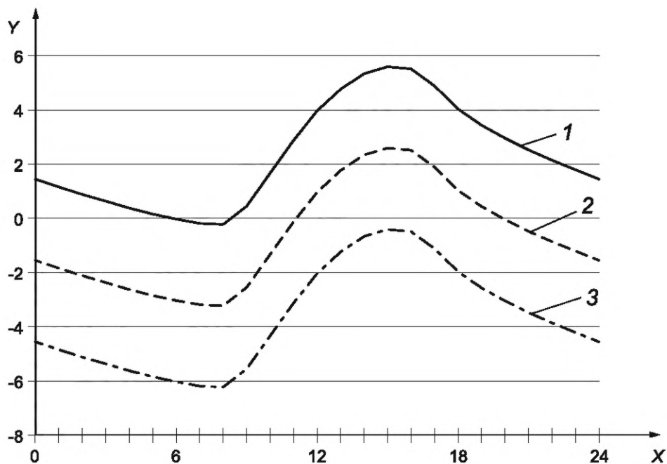
X — время, ч; Y — температура, °C; 1 — линия верхнего предела температуры 3 °C; 2 — линия средней температуры; 3 — линия нижнего предела температуры -3 °C
