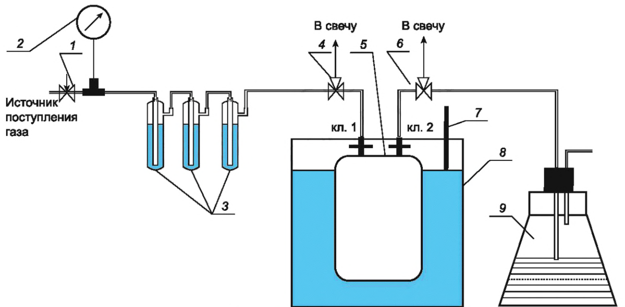
1 — газовый редуктор/выход газопровода; 2 — манометр газового редуктора; 3 — увлажнитель газа; 4, 6 — краны соединительные трехходовые; 5 — calorиметрическая бомба; 7 — средство измерения температуры; 8 — термостат; 9 — склянка (счетчик пузырьков)
