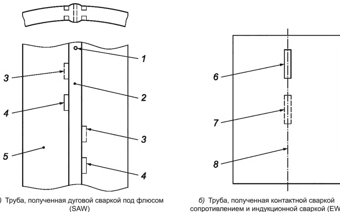
а) Труба, полученная дуговой сваркой под флюсом (SAW) б) Труба, полученная контактной сваркой сопротивлением и индукционной сваркой (EW) 1 — сквозное настроечное отверстие; 2 — сварной шов, полученный дуговой сваркой под флюсом; 3 и 7 — продольные внутренние настроечные пазы; 4 и 6 — продольные наружные настроечные пазы; 5 — настроечный образец-труба; 8 — осевая линия сварного шва
