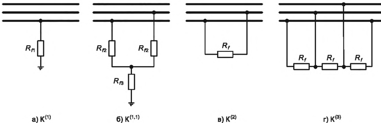
Рисунок А.5 — Подключение переходного сопротивления в месте повреждения
