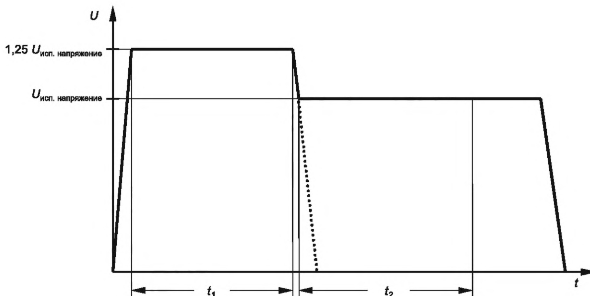
Рисунок 3 — Испытательные напряжения
