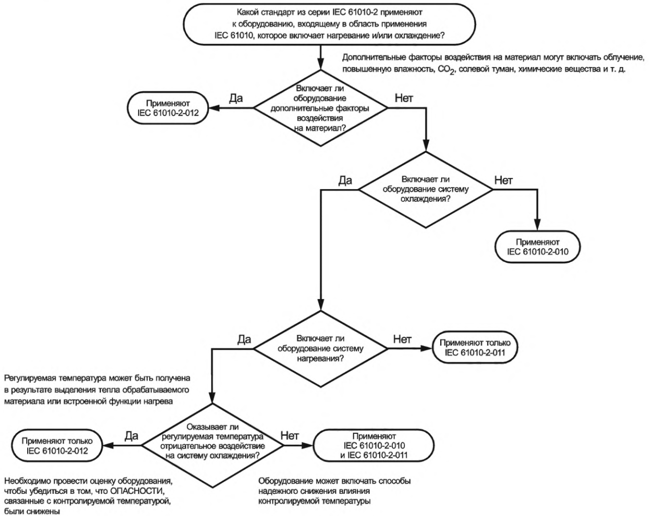
Рисунок 102 — Схема последовательности операций процесса выбора
