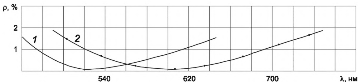
Рисунок А.6 — Коэффициент отражения от поверхности стекол марок СТК9, СТК19 с двухслойным покрытием (51P×0,26).(43P×1,24).350
