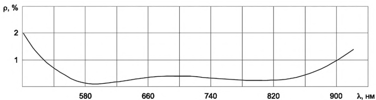
Рисунок А.18 — Коэффициент отражения от поверхности стекла марки ОФ6 с трехслойным покрытием 45P.(44P×2).43P.350
