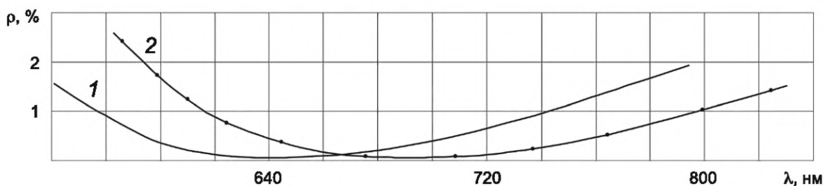
Рисунок А.9 — Коэффициент отражения от поверхности стекол марок ФК14, ФК13, ФК24, ФК11 с двухслойным покрытием (44P×0,44).(43P×1,24).350
