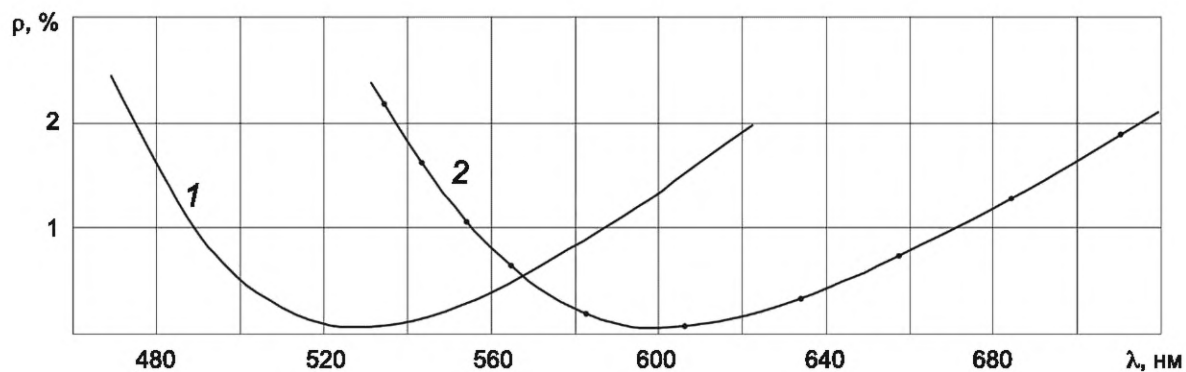
Рисунок А.10 — Коэффициент отражения от поверхности стекла марки ОК1 с двухслойным покрытием (44P×0,44).(43P×1,24).350
