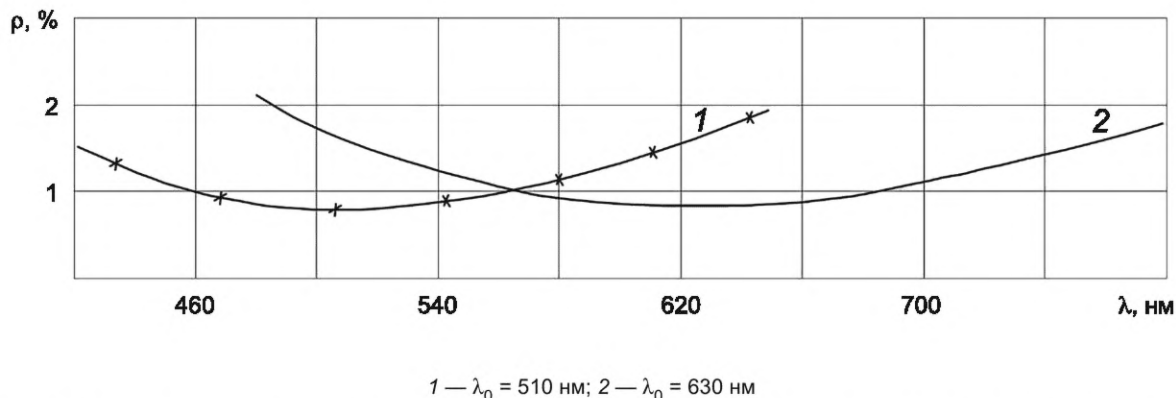
Рисунок А.3 — Коэффициент отражения от поверхности стекол марок СТК9, СТК19 с покрытием 43P.350
