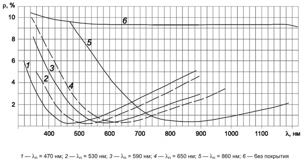
Рисунок А.4 — Коэффициент отражения от поверхности стекла марки ТБФ8 с покрытием 43P.350
