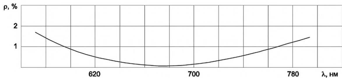
Рисунок А.8 — Коэффициент отражения от поверхности стекла марки ОФ4 с двухслойным покрытием (44P×0,44).(43P×1,24).350
