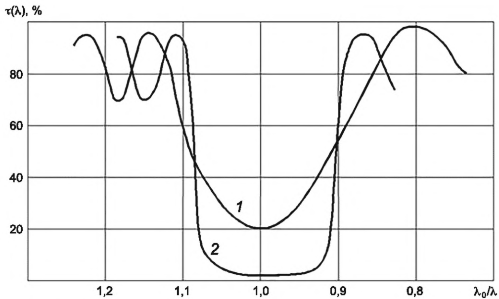
Рисунок Б.4 — Спектральные кривые коэффициентов отражения (кривая 1) и пропускания (кривая 2) просветляющего покрытия (39I:37I) \times m:39I, где m = 2 (кривая 1) и m = 8 (кривая 2) на деталях из фтористого кальция
