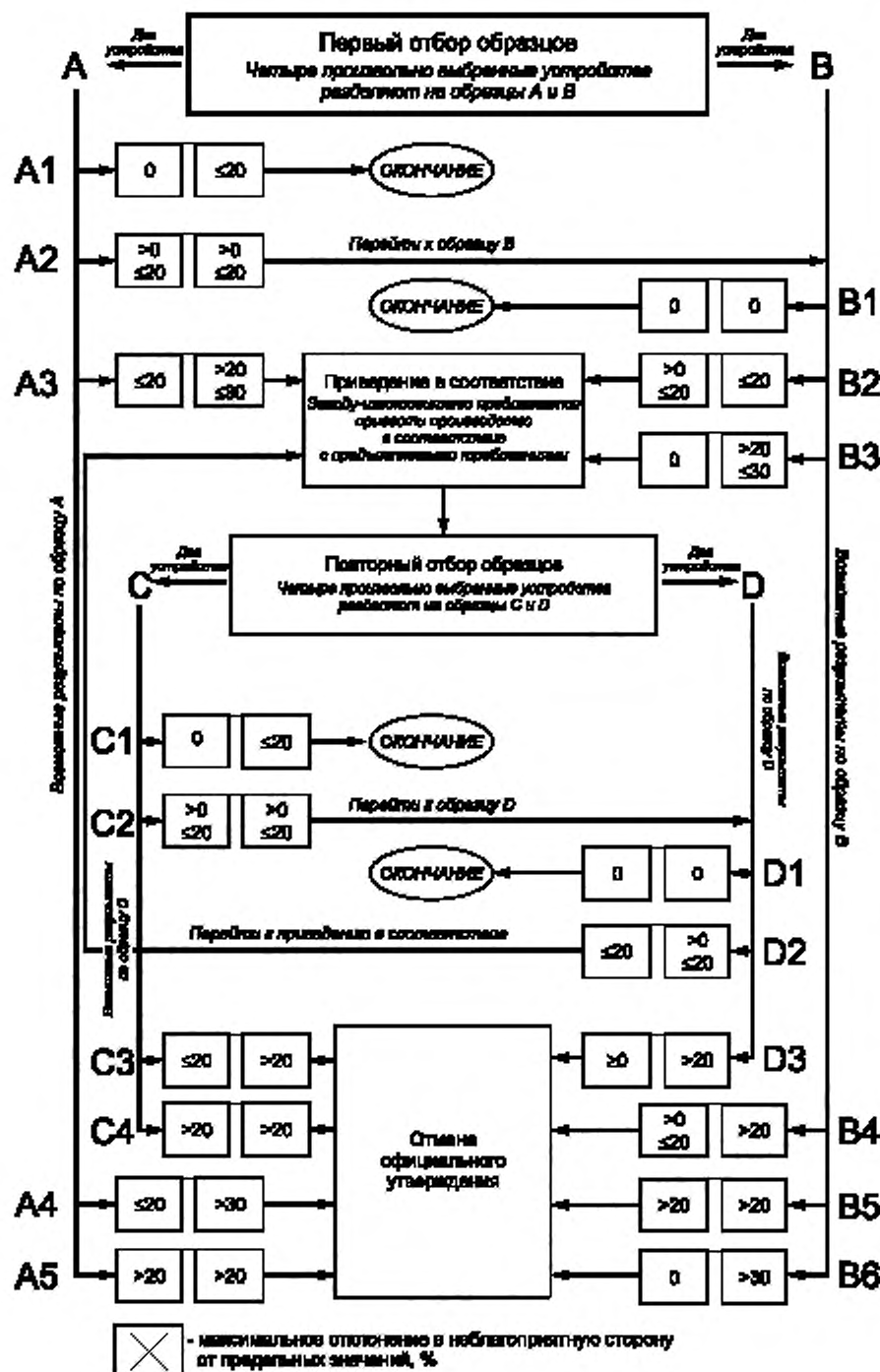
Рисунок 1 — Схема проведения процедуры отбора образцов
