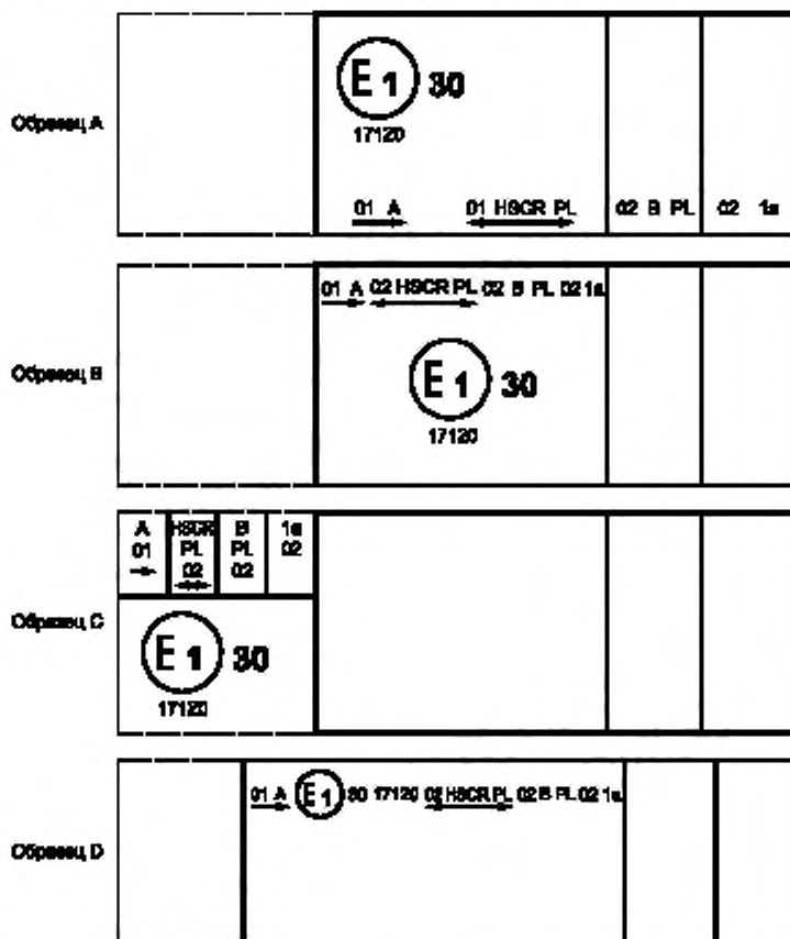
Рисунок 8 — Упрощенная маркировка сгруппированных, комбинированных или совмещенных огней
